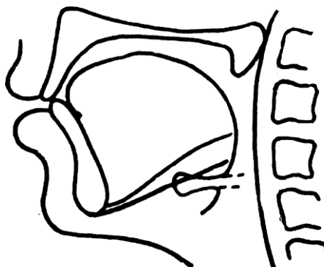
Расми 1.4.23 - Нақшаи рентгенограммаи овози “ч”
