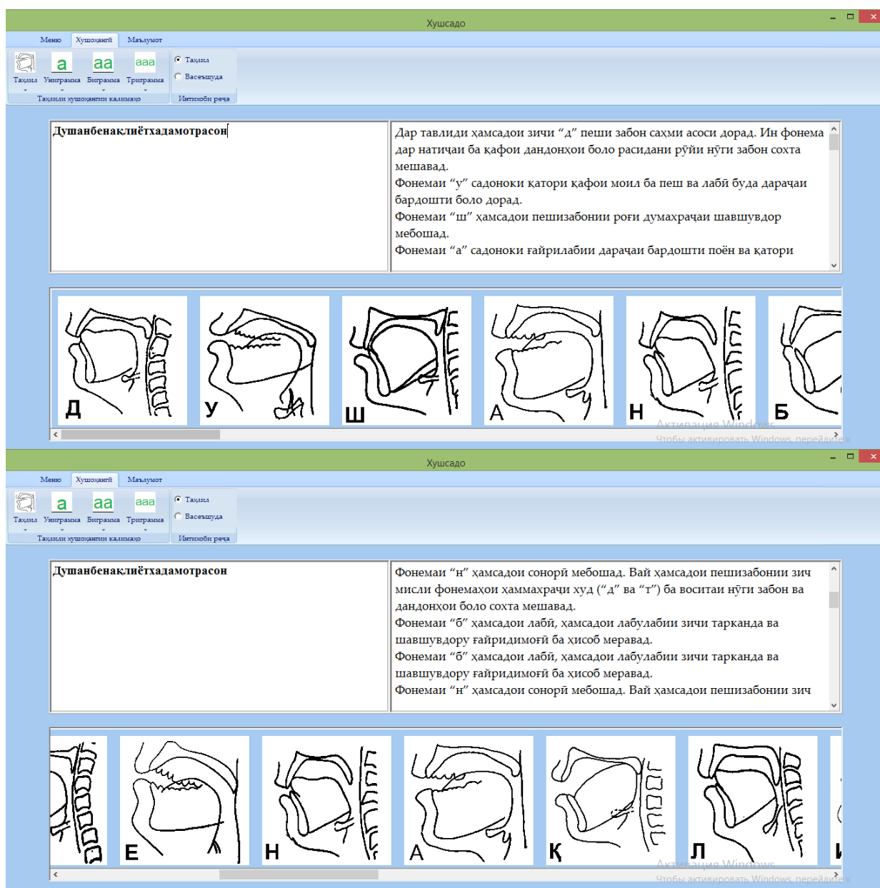
Расми 3.3.2 - Таҳлили хусусиятҳои овозҳои калимаи “Душанбенақлиётҳадамотрасон”
