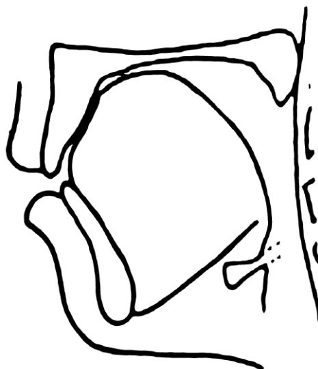
Расми 1.4.26 - Нақшаи рентгенограммаи овози “й”
