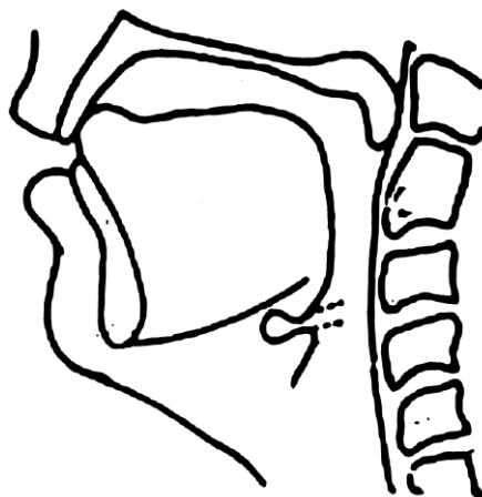
Расми 1.4.15 - Нақшаи рентгенограмми овози “д”
