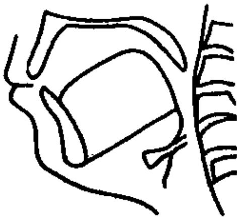
Расми 1.4.12 - Нақшаи рентгенограммаи овози “м”
