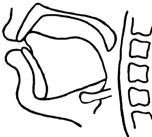
Расми 1.4.25 - Нақшаи рентгенограммаи овози “р”
