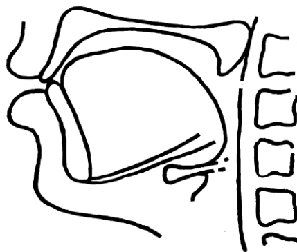
Расми 1.4.22 - Нақшаи рентгенограммаи овози “ш”
