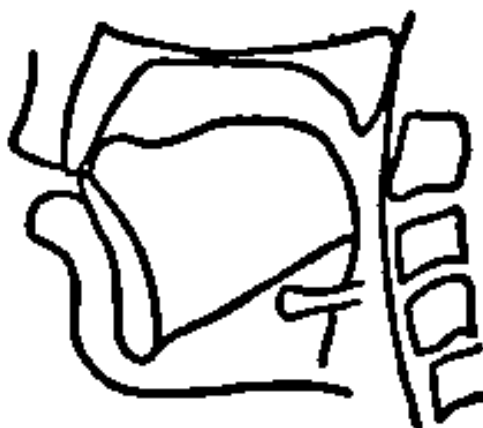
Расми 1.4.19 - Нақшаи рентгенограммаи овози “с”
