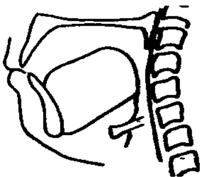
Расми 1.4.10 - Нақшаи рентгенограммаи овози “б”
