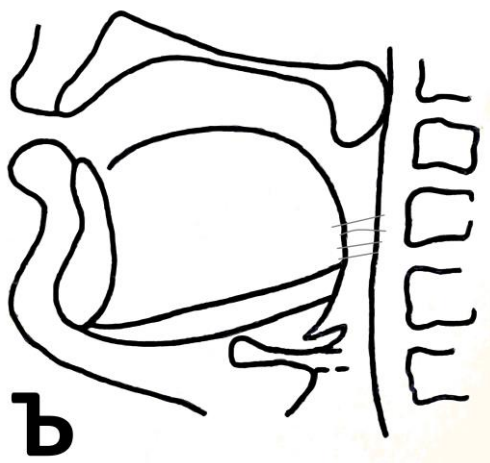
Расми 1.4.32 - Нақшаи рентгенограммаи овози “Ъ”
