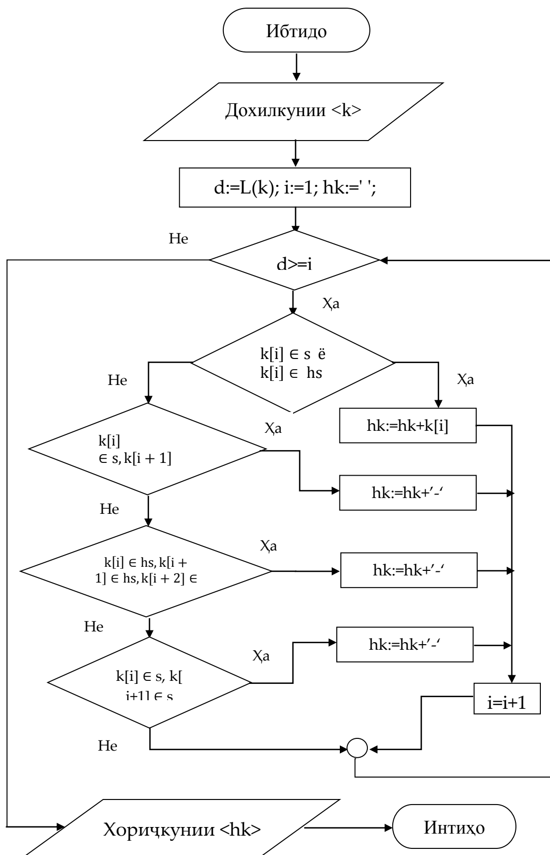
Расми 3.1.2 - Блок-схемаи ба ҳиҷоҳо ҷудокунии калимаҳои тоҷикӣ
