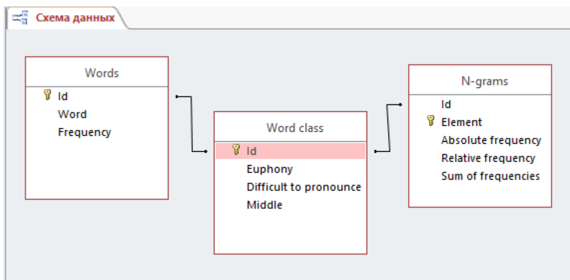
Расми 3.1.4 - Сохтори ҷадвалҳои пойгоҳи додаҳо
