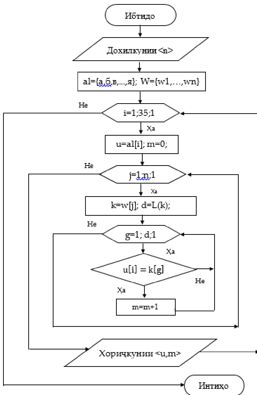
Расми 3.1.1 - Блок-схемаи коркарди униграммаҳои калимашаклҳои
