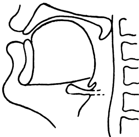
Расми 1.4.24 - Нақшаи рентгенограммаи овози “ч”
