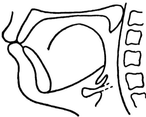
Расми 1.4.13 - Нақшаи рентгенограммаи овози “в”
