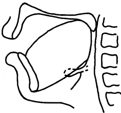
Расми 1.4.30 - Нақшаи рентгенограммаи овози “х”
