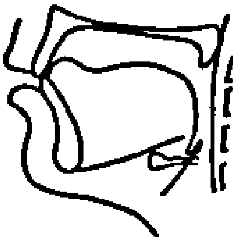
Расми 1.4.18 - Нақшаи рентгенограммаи овози “з”
