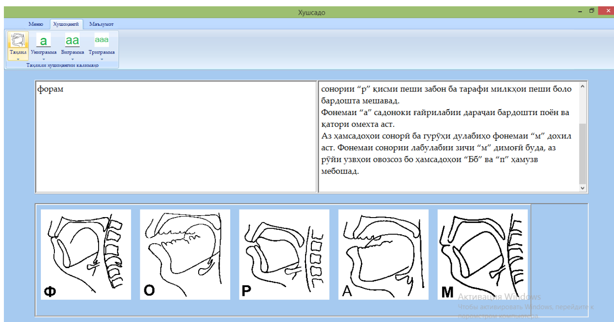
Расми 3.3.1 - Таҳлили хусусиятҳои овозҳои калимаи ФОРАМ
