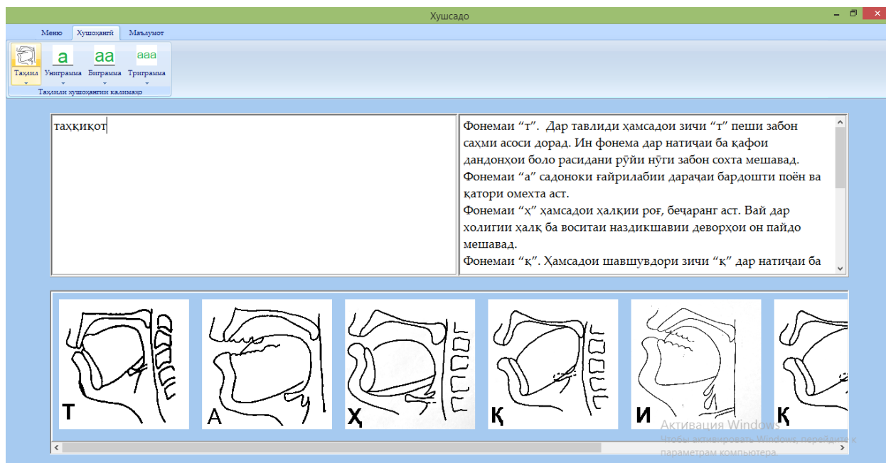
Расми 3.3.3 - Таҳлили хусусиятҳои овозҳои калимаи ТАҲҚИҚ
