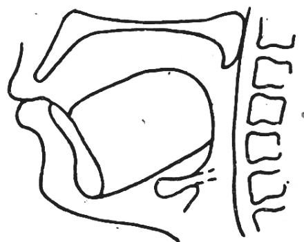
Расми 1.4.11 - Нақшаи рентгенограммаи овози “п”
