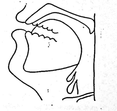
Расми 1.4.5 - Нақшаи рентгенограммаи овози “и”
