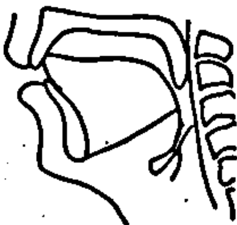
Расми 1.4.20 - Нақшаи рентгенограммаи овози “л”
