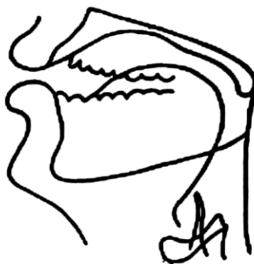
Расми 1.4.7 - Нақшаи рентгенограммаи овози “у”
