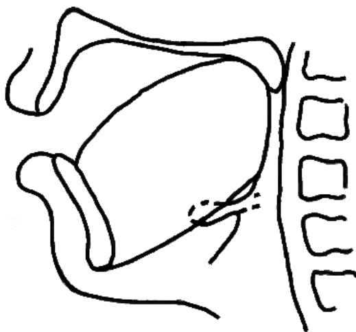
Расми 1.4.31 - Нақшаи рентгенограммаи овози “қ”
