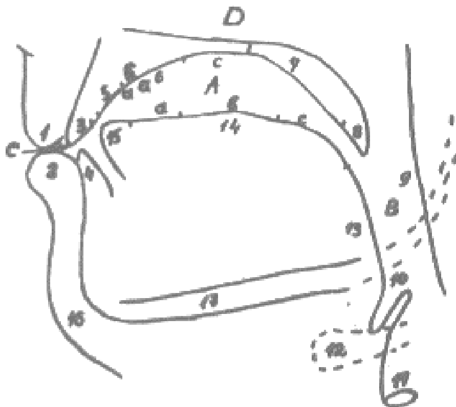
Расми 1.4.1 - Инъикоси узвҳои нутқ дар рентгенограмма
