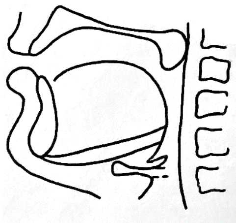
Расми 1.4.33 - Нақшаи рентгенограммаи овози “ҳ”
